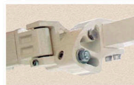
Supports de bras permettant un réglage facile et rapide de l'inclinaison (5° à 45°).
